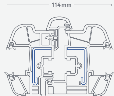
Arcade organisch Stulpausführung Abb.: 1:2,5
