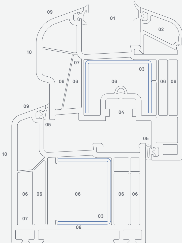
Arcade organisch Abb.: 1:1
